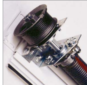
Yay Kırılma Emniyet Sistemi
